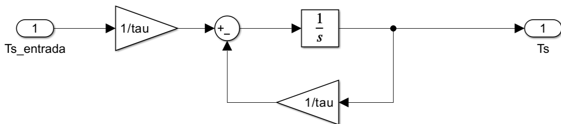
Figura 65: Sensor de temperatura
