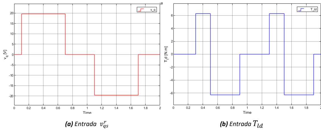
Figura 14: Entrada de tensión y torque de perturbación
