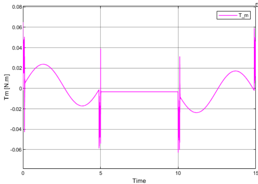
Figura 98: Torque T_m con controlador discreto
