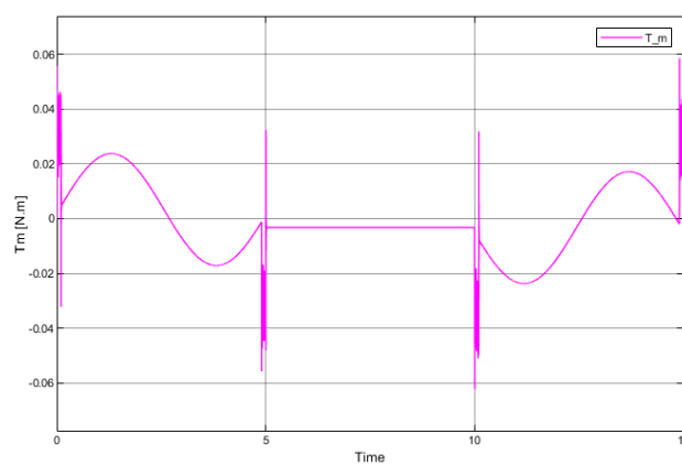
Figura 102: Torque T_m con controlador discreto codificado
