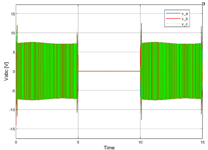
Figura 85: Curvas de v_{abc} con \omega_{n\_modulador} = 18000 \text{ rad/s}
