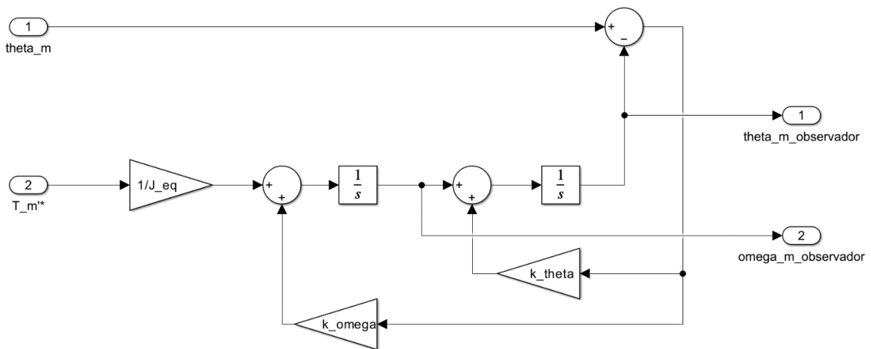
Figura 38: Observador de orden reducido
