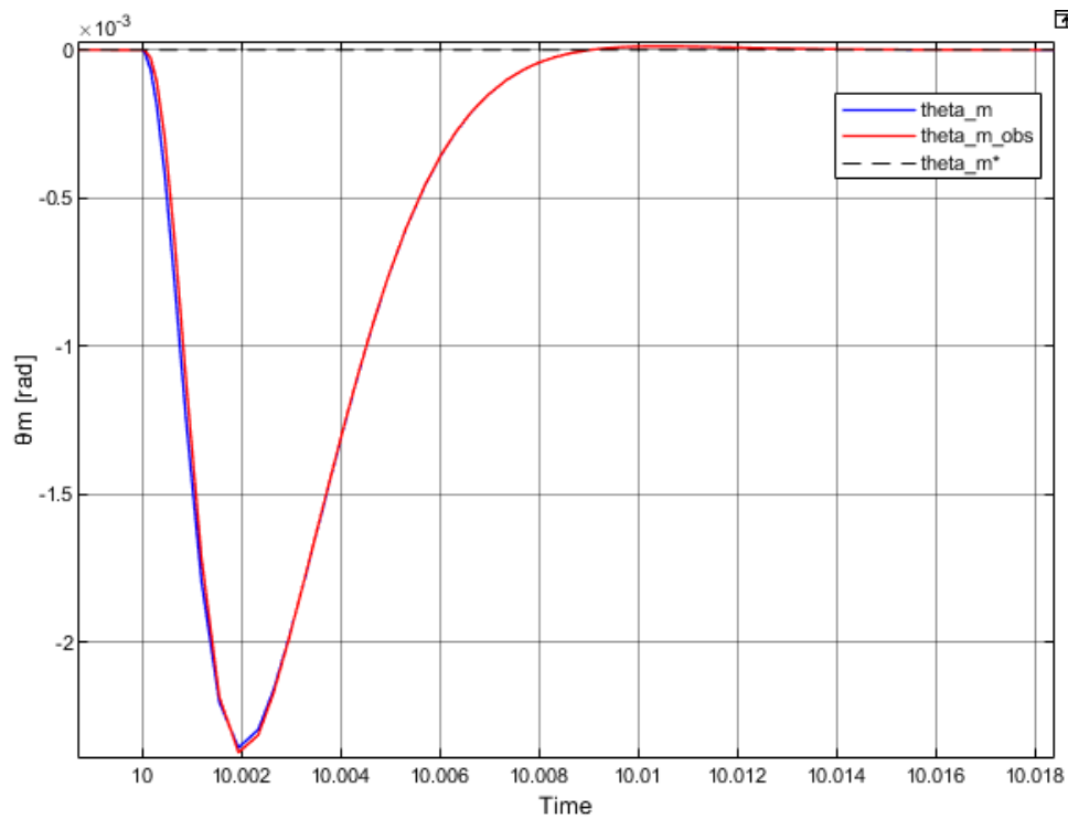
Figura 60: Posición con \theta_m(t) observador de estados con acción integral. Detalle en t = 10 s.
