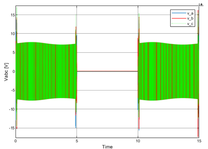
Figura 97: Curvas de tensiones v_{abc} con controlador discreto
