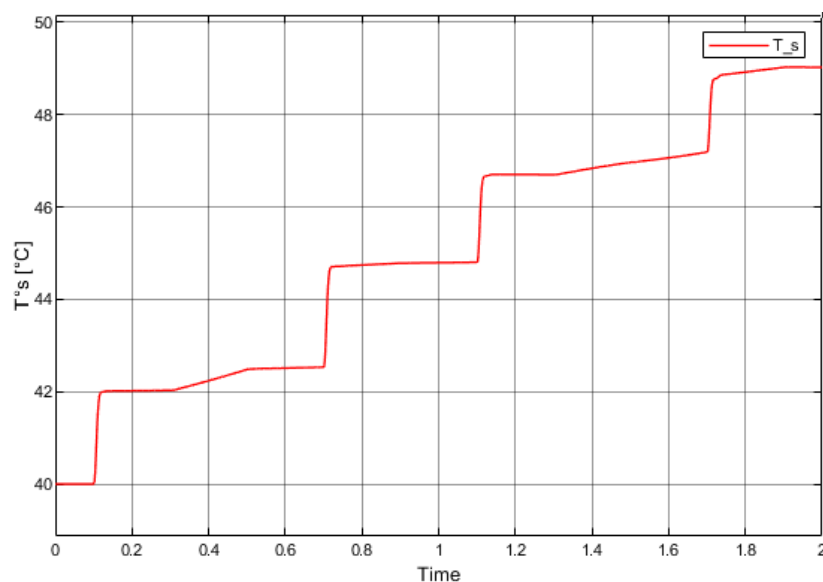
Figura 20: Temperatura T_s
