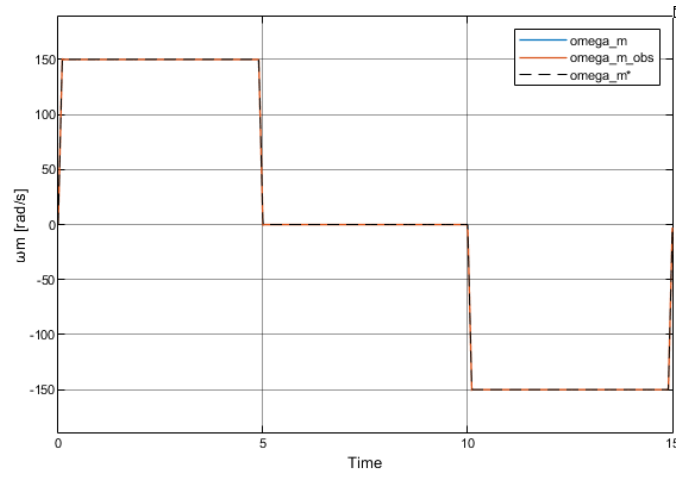
Figura 52: Velocidad angular real vs observada vs consigna
