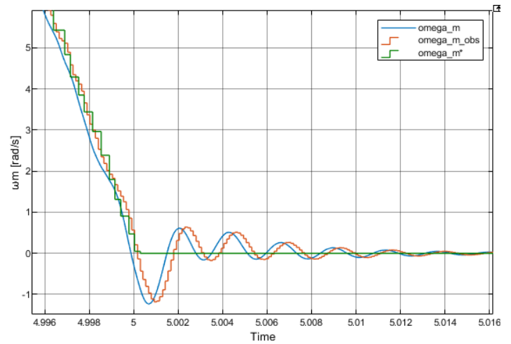
Figura 95: Curvas de velocidad \omega_m con controlador discreto
