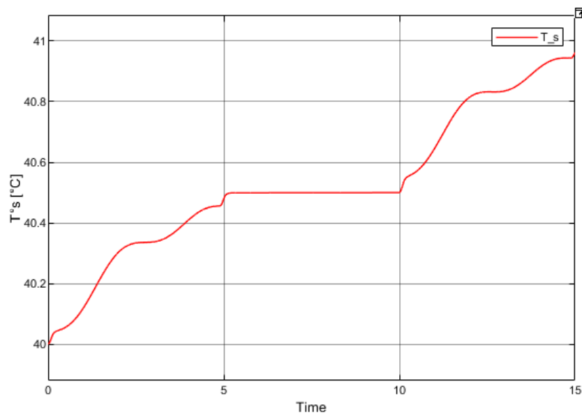
Figura 76: Curva de temperatura con \tau = 0.05 \text{ s}
