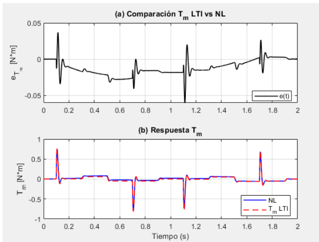
Figura 23: Comparación T_m para LTI y NL
