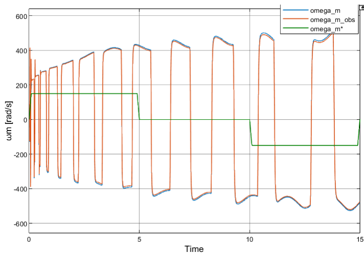
Figura 82: Curvas de velocidad con \omega_{n\_modulador} = 6000 \text{ rad/s}
