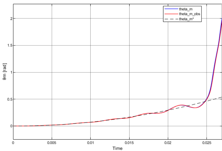
Figura 67: Curvas de posición con \omega_{n_{pos}} = 2000 \text{ rad/s}
