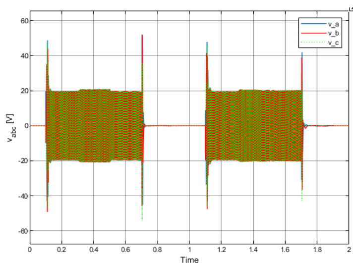
Figura 17: Tensiones v_{abc}
