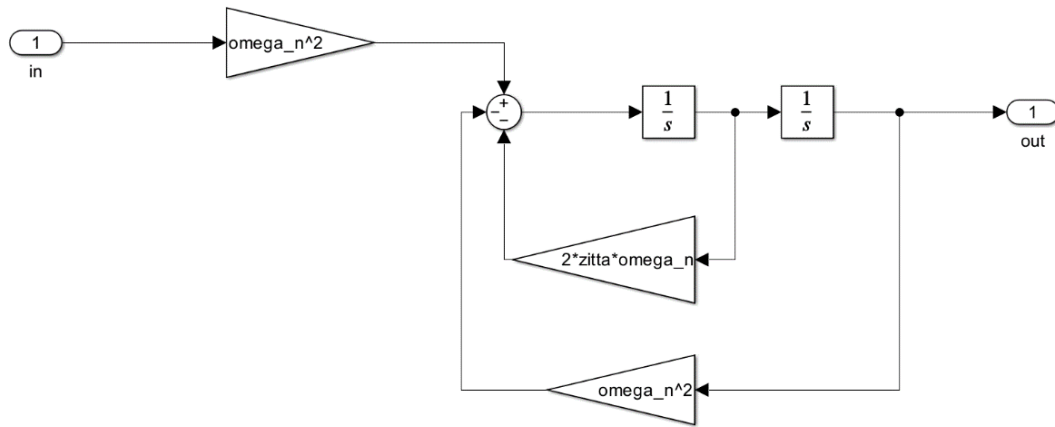
Figura 64: Sensor no ideal genérico
