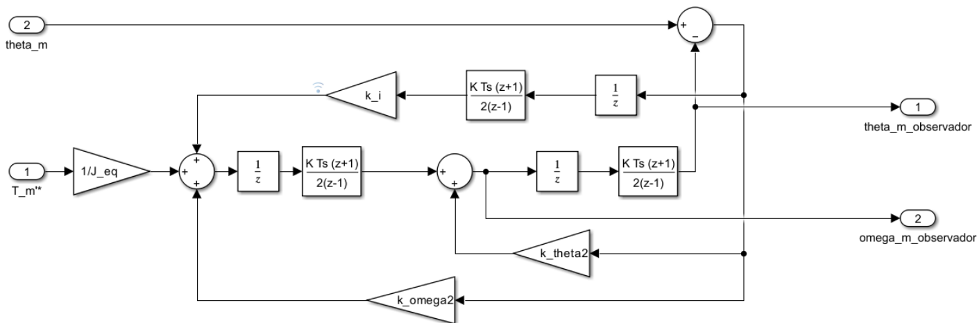
Figura 92: Observador aumentado discretizado
