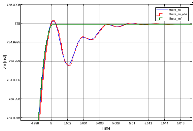
Figura 100: Curvas de posición \theta_m controlador discreto codificado
