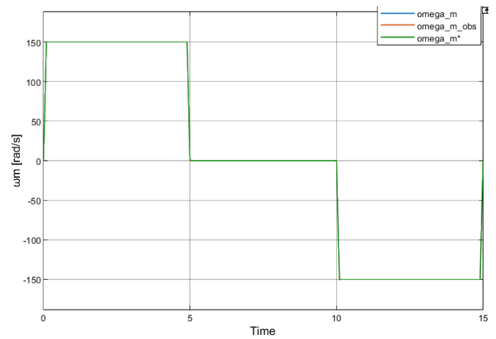
Figura 83: Curvas de velocidad con \omega_{n\_modulador} = 18000 \text{ rad/s}
