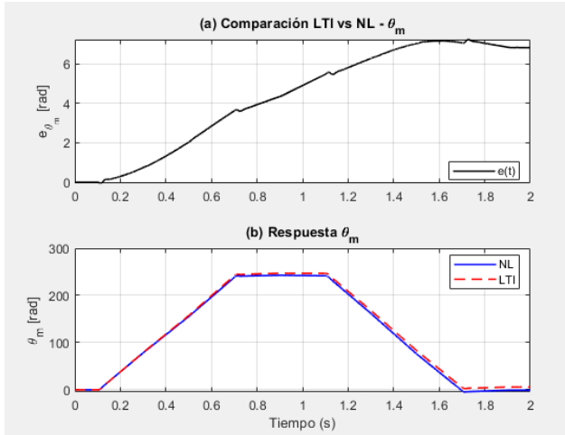
Figura 21: Comparación \theta_m para LTI y NL
