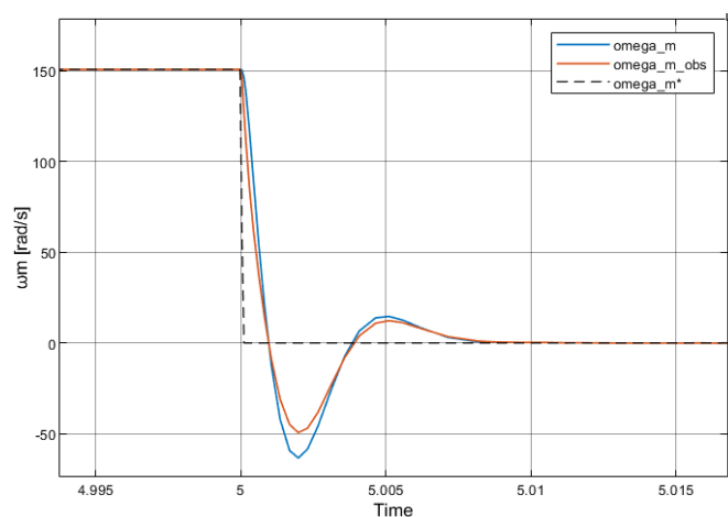
Figura 44: Detalle en t = 5s
