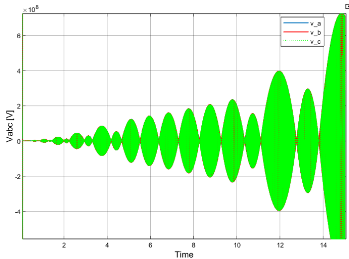
Figura 84: Curvas de v_{abc} con \omega_{n\_modulador} = 6000 \text{ rad/s}
