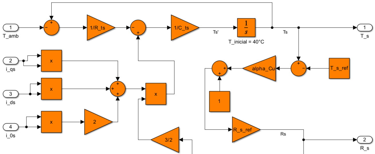
Figura 5: Subsistema térmico
