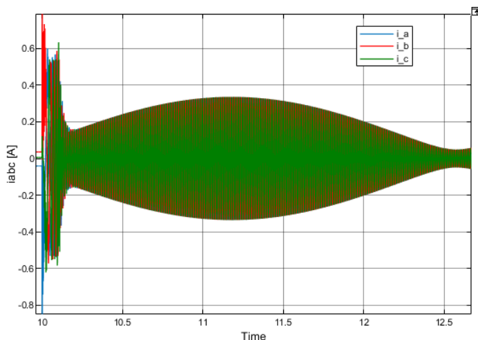
Figura 77: Curvas de corriente con \omega_{n\_corriente} = 12000 \text{ rad/s}
