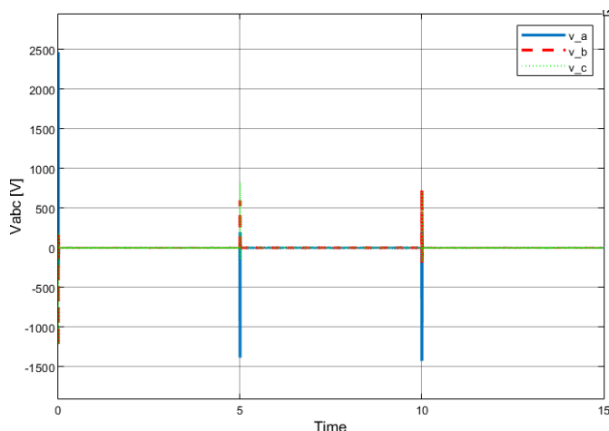
Figura 47: Tensiones v_{abc}(t)
