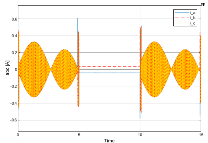
Figura 56: Corrientes i_{abc}
