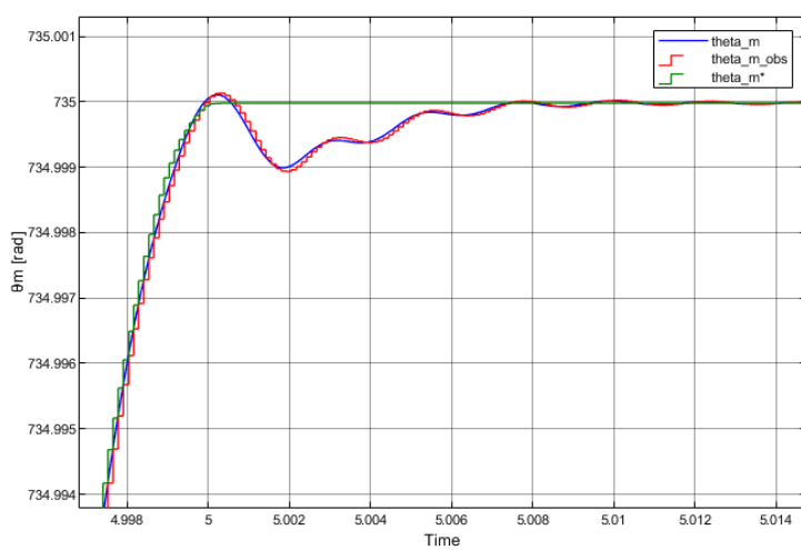
Figura 94: Curvas de posición \theta_m con controlador discreto
