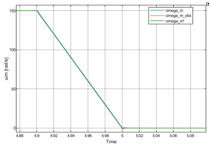
Figura 73: Curvas de velocidad con \omega_{n\_pos} = 6000 \text{ rad/s}
