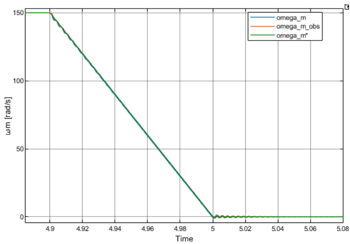
Figura 72: Curvas de velocidad con \omega_{n\_pos} = 4000 \text{ rad/s}
