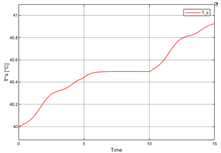
Figura 75: Curva de temperatura con \tau = 0.5 \text{ s}
