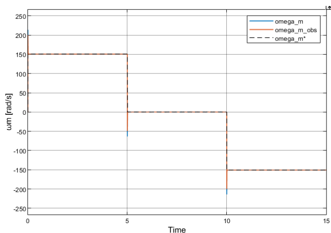
Figura 43: Comparación \omega_m(t) , \omega_m^*(t) y observador
