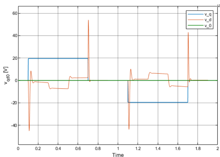
Figura 16: Tensiones v_{qd0}
