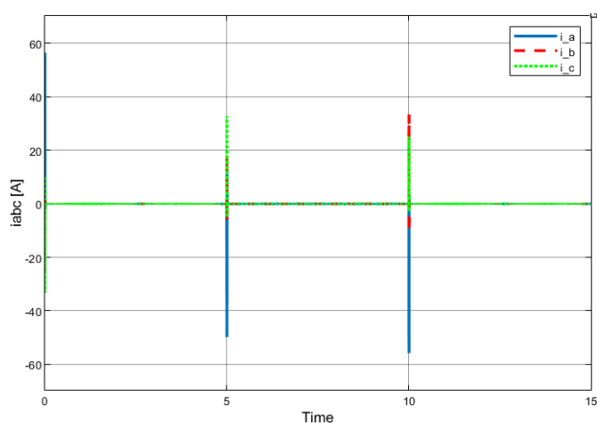
Figura 46: Corrientes i_{abc}(t)
